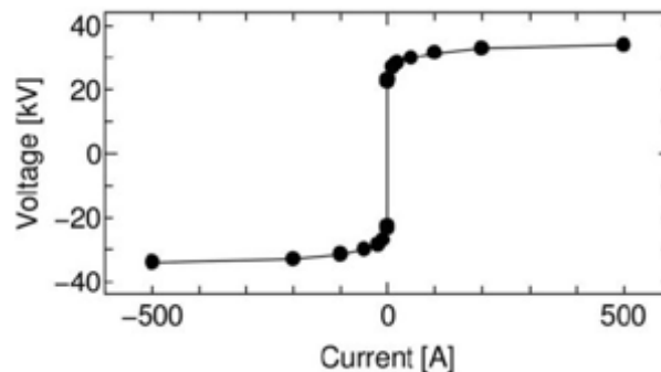
Fig. 4. Curva característica V-I del descargador empleado. Fuente: [20].
