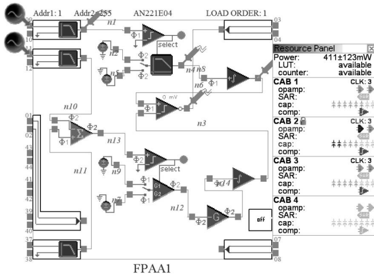
Fig. 2. Ilustración interfaz de programación gráfica para dispositivo de proceso.
