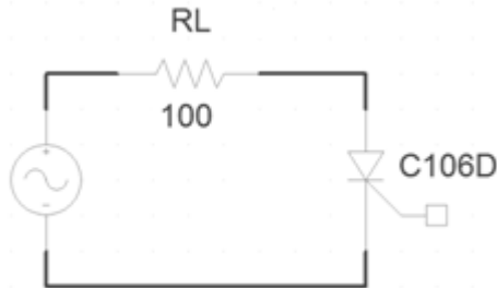
Fig. 3. Diagrama esquemático para rectificador controlado por disparo de SCR. Fuente: Autores
